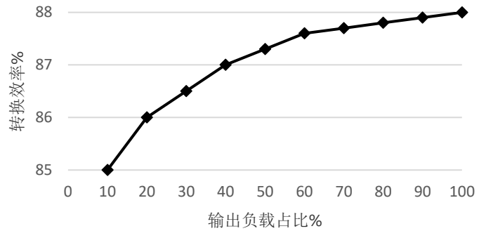
负载效率曲线
