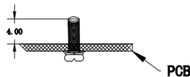
标准型 61*57.9*12.7mm
