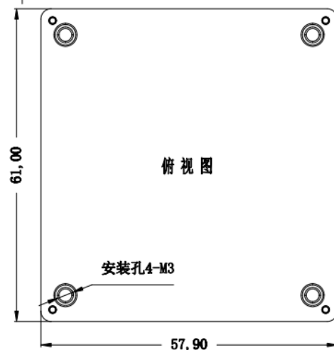
标准型 61*57.9*12.7mm
