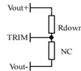
电压下调: 在Trim和输出正之间增加电阻Rdown
