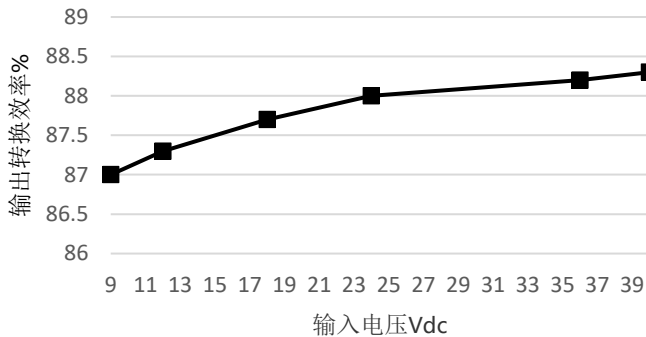
输入电压效率曲线
